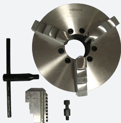
Патрон токарный HORTZ комплект
